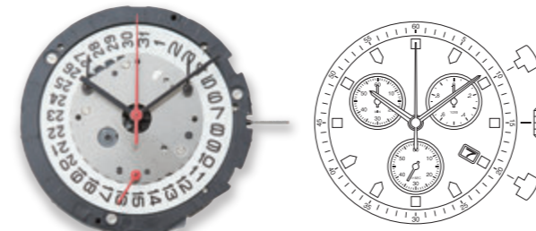
6S30 厚度 4.90 毫米 计时 (分 / 秒) / 1/20 秒 电池寿命四年 (SR927W)
