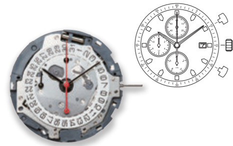
OS60 厚度 4.13 毫米 计时 (时 / 分 / 秒) / 1/20 秒 电池寿命二年 (SR927W)
