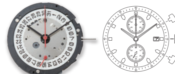
6S11 厚度 4.90 毫米 计时 (分 / 秒) 电池寿命四年 (SR927W)
