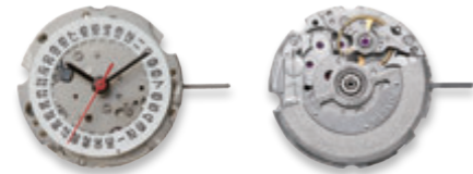
6T15 厚度 5.98 毫米 / 21 钻 频率 28800 次 / 小时 自动上条 / 手动上条 快速日历设定
